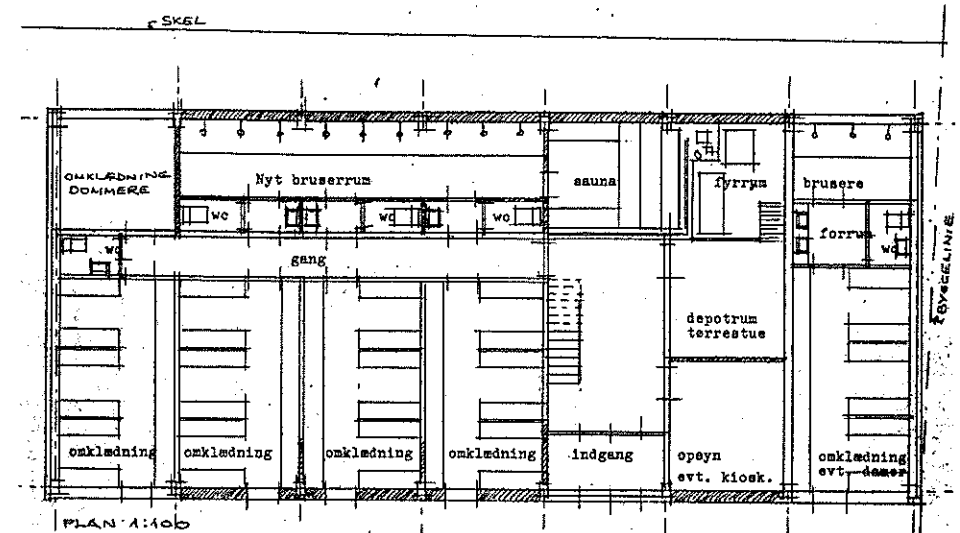
PLAN 1:100
